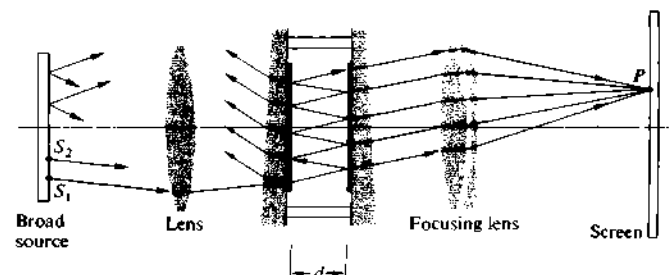
Figure 9.43 Fabry-Perot etalon.
