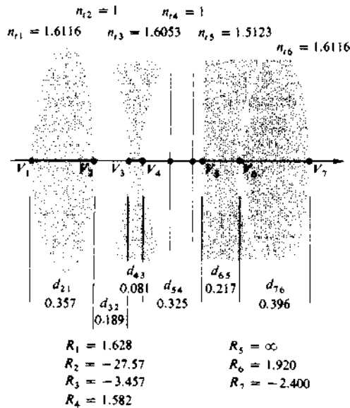
Figure 6.10 A Tessar.
