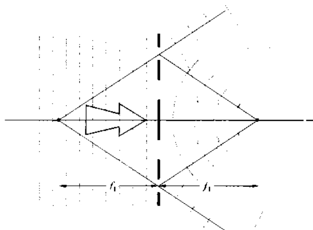
Figure 10.48 Zone-plate foci.
