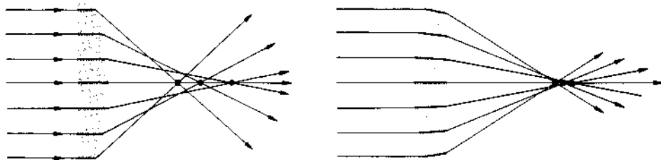
Figure 6.16 SA for a planar-convex lens.
